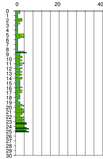
Rif. :GualcoSrl n° 4 quota inizio: p.c.
