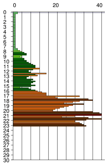
Rif. :GualcoSrl n° 6 quota inizio: p.c.
